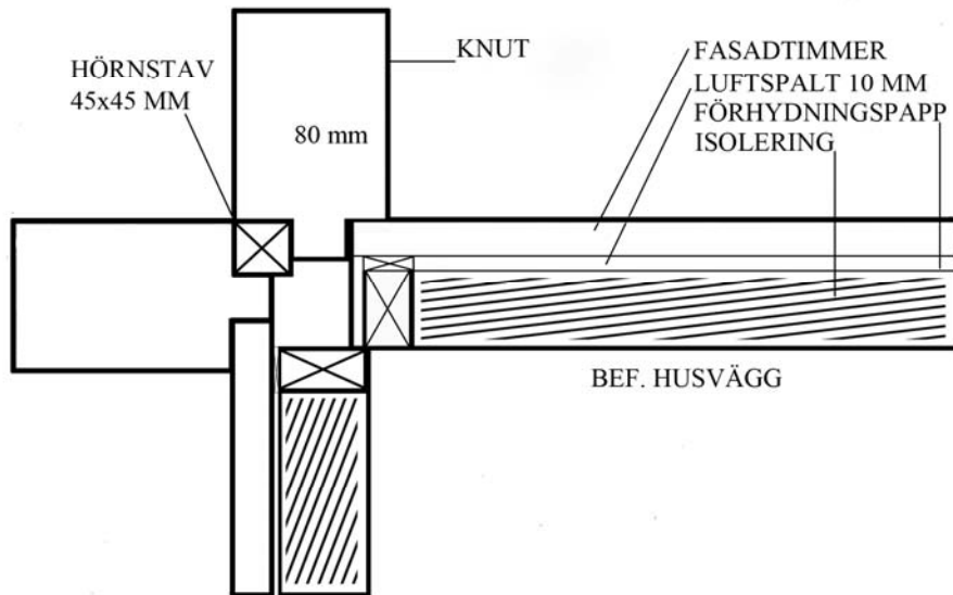
FASADHÖRN 1:5
