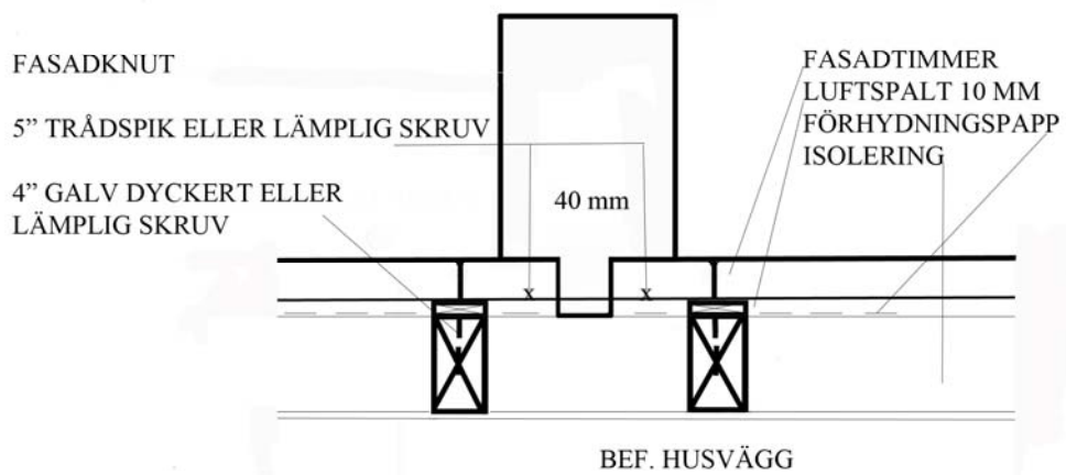
DETALJ AV KNUT MITT PÅ VÄGG 1:5
